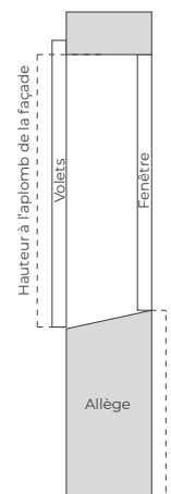
Appui droit (non débordant) solution SA et BSA
