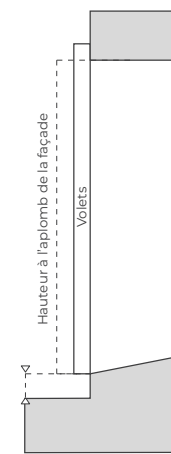
Porte-fenêtre avec marche solution BSA
