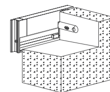
Détail solutions SA et BSA
