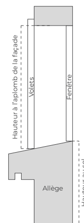
Appui fenêtre solution AA
