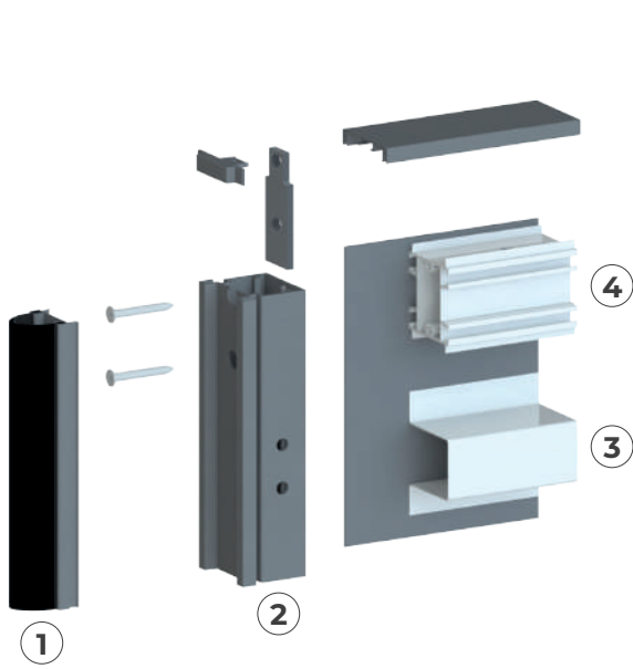
Rail inox de coulissant en U anti-déraillement
