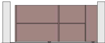
Quadra C7 2 caissons si H ≤ 1440 mm
